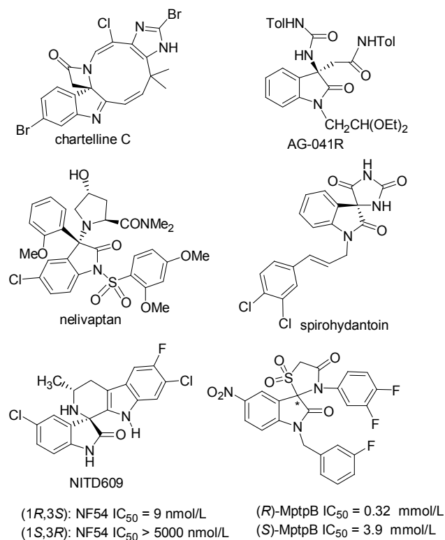
图1 一些代表性的具有胺基季碳氧化吲哚结构的生物活性分子 Figure 1 Some representative bioactive aminooxindole derivatives
